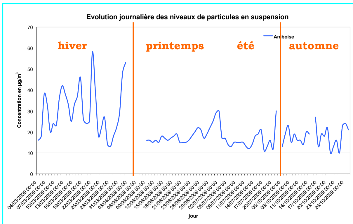
Graphe 3 : évolution journalière des particules en suspension à Amboise en 2009
