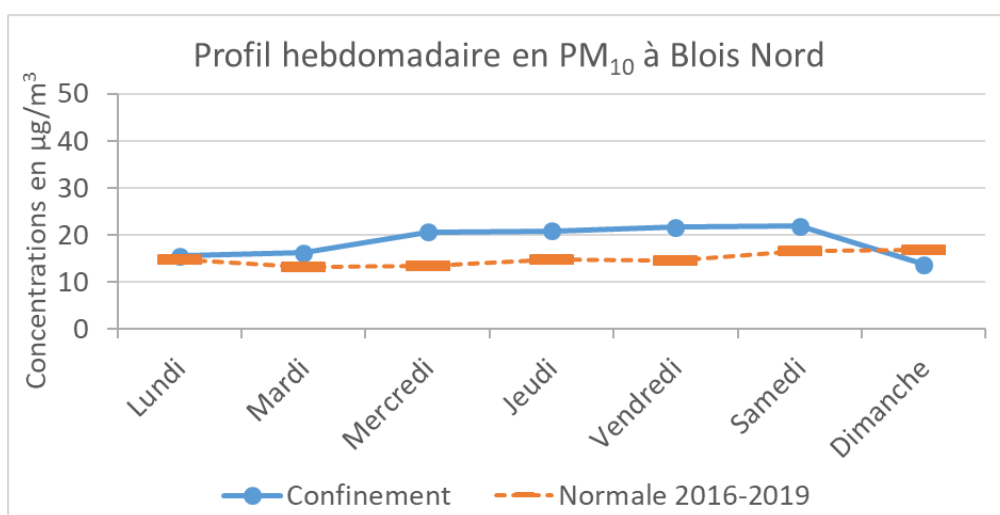
Figure 5 : Profils hebdomadaires en en particules en suspension (PM 10 ) sur le site urbain de fond de Blois Nord à Blois
