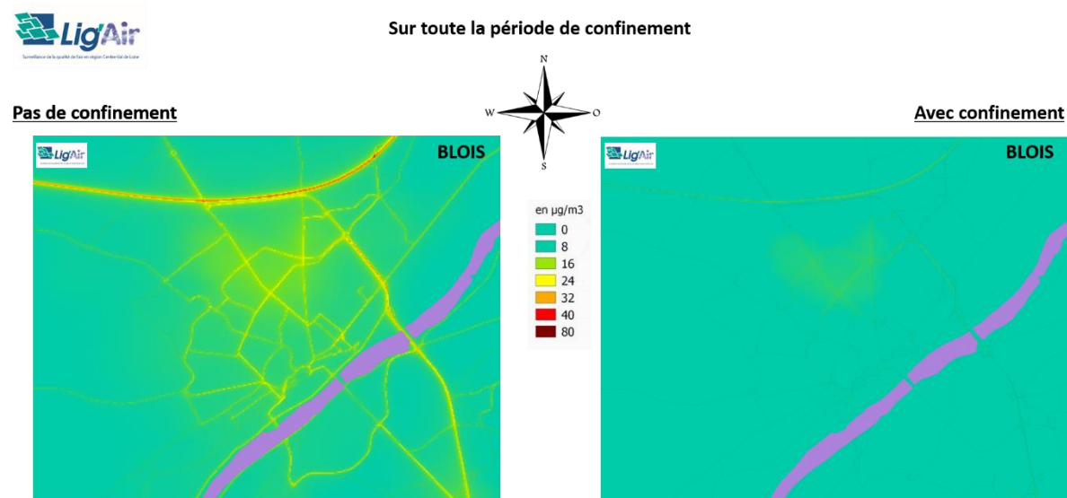
Figure 8 : Evolution spatiale des concentrations moyennes en NO 2 sur Blois Agglopolys (concentrations moyennes simulées sur la période du 18 mars au 10 mai 2020 suivant les deux situations (« sans confinement » et « avec confinement »))
