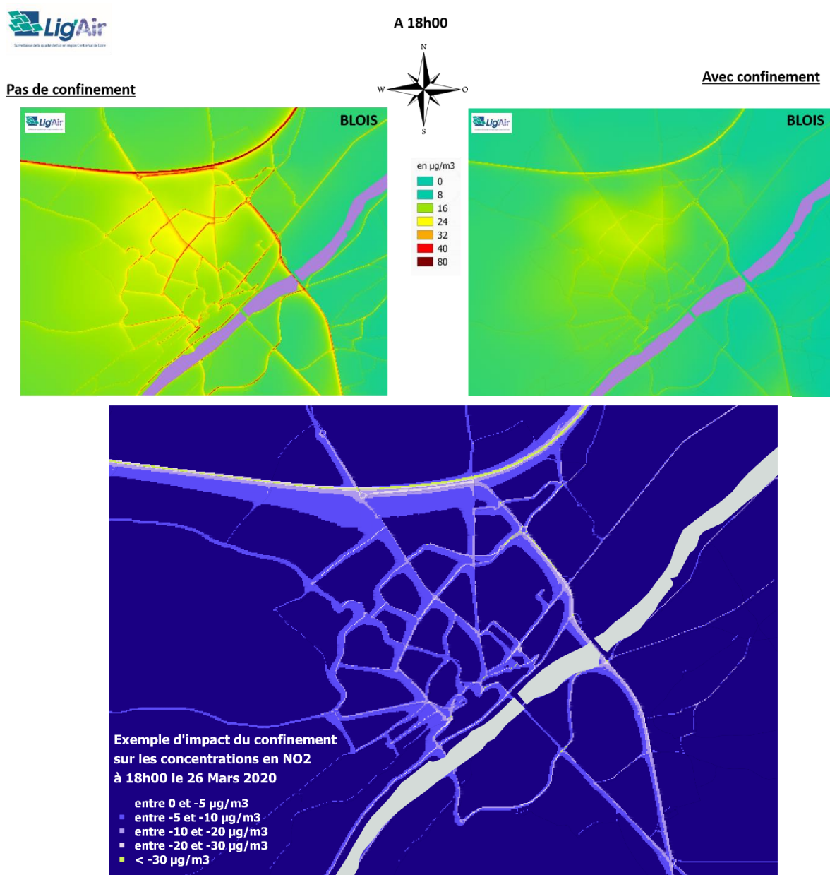
Figure 9 : Concentrations horaires en NO 2 obtenues à 18h00 le Jeudi 26 mars (a) sans confinement et (b) pendant le confinement et (c) carte de différence, sur le territoire de Blois Agglopolys
