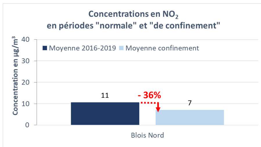
Figure 1 : comparaison des concentrations moyennes en dioxyde d'azote (NO 2 ) sur l'agglomération blésoise durant le confinement et en période « normale »
