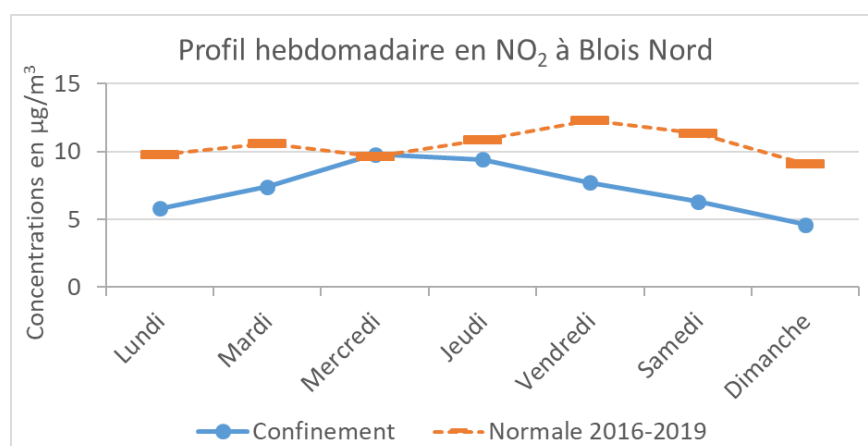
Figure 2 : Profils hebdomadaires en dioxyde d'azote (NO 2 ) sur le site urbain de fond de Blois Nord
