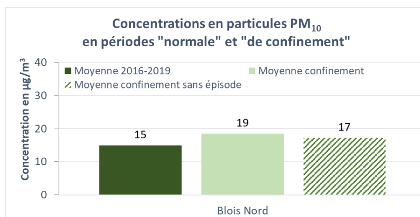
Figure 4 : comparaison des concentrations moyennes en particules en suspension (PM 10 ) sur l'agglomération blésoise durant le confinement et en période « normale »
