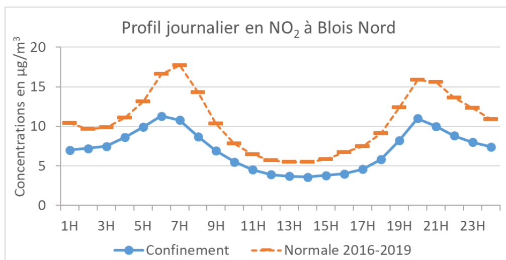
Figure 3 : Profils journaliers en dioxyde d'azote (NO 2 ) sur le site urbaine de fond de Blois Nord
